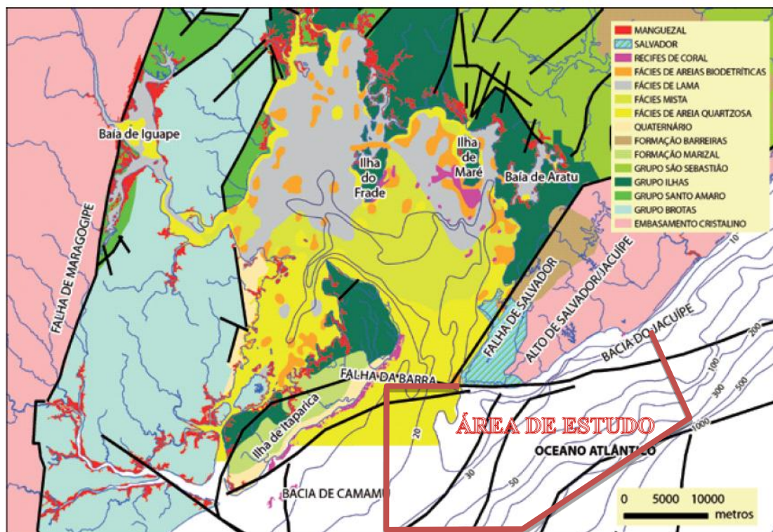
Fig. 4. Geologia do entorno da área de estudo (modificada de Dominguez e Bittencourt, 2009).
