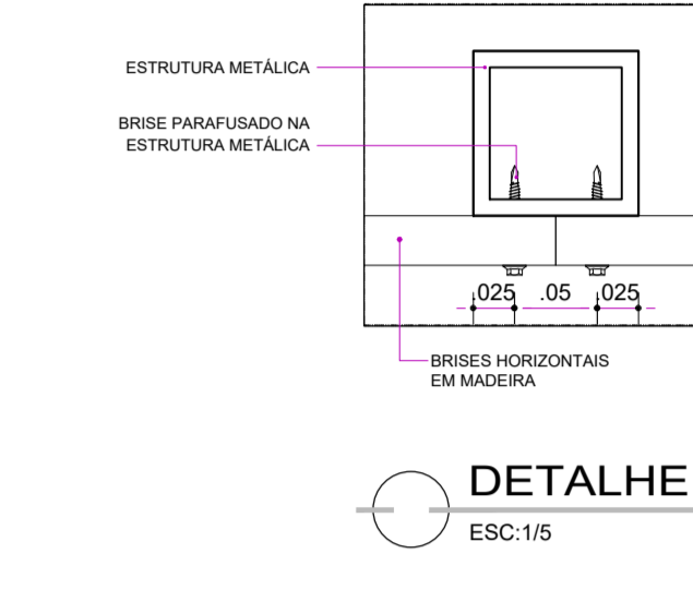
DETALHE 02 ESC. 1/5
