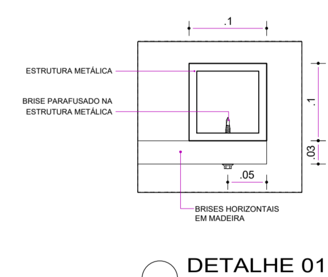
DETALHE 01 ESC. 1/5
