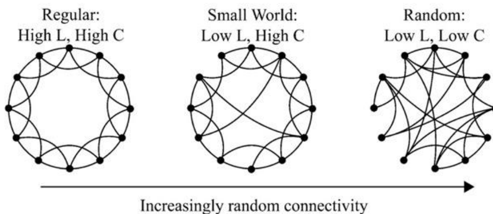
Figura 17: Diagrama ilustrativo do modelo de Watts demonstrando que as redes de mundo-pequeno ocorrem a meio caminho do processo de aleatorização de redes regulares.
