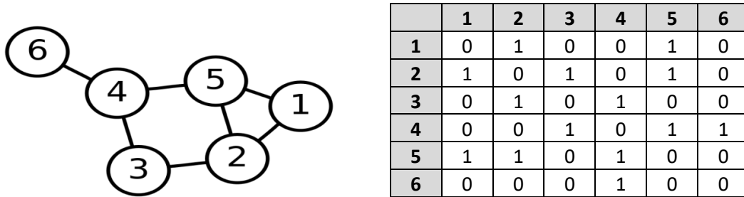
Figura 7: Esquemática de uma rede simples com matriz de adjacência correspondente ao lado.
