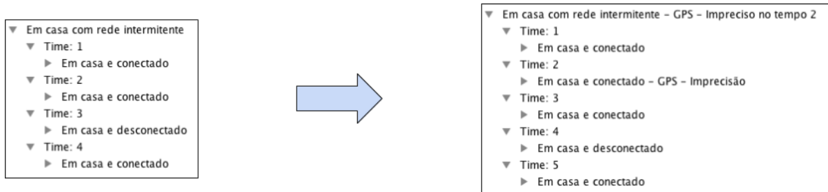
Figura 3.24 Exemplo de transformação de uma situação com o padrão de defeito Granularidade Incompatível/Imprecisão no tempo 2, o qual reflete uma imprecisão no sensor GPS após a leitura ocorrida no tempo 1.
