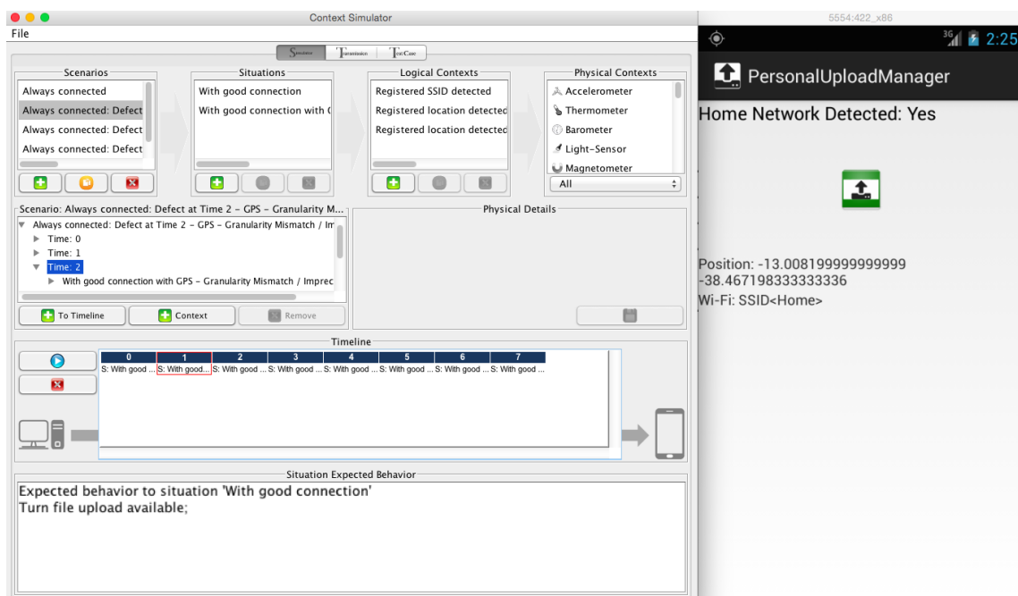
Figura 3.33 Aplicação sob teste funcionando corretamente com o contexto do usuário coincidindo com localização e conectividade configuradas na aplicação.
