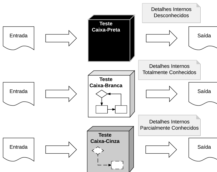
Figura 2.1 Diferença no nível de conhecimento exigido pelo testador em relação à aplicação entre o teste de caixa-preta, caixa-branca e caixa-cinza.
