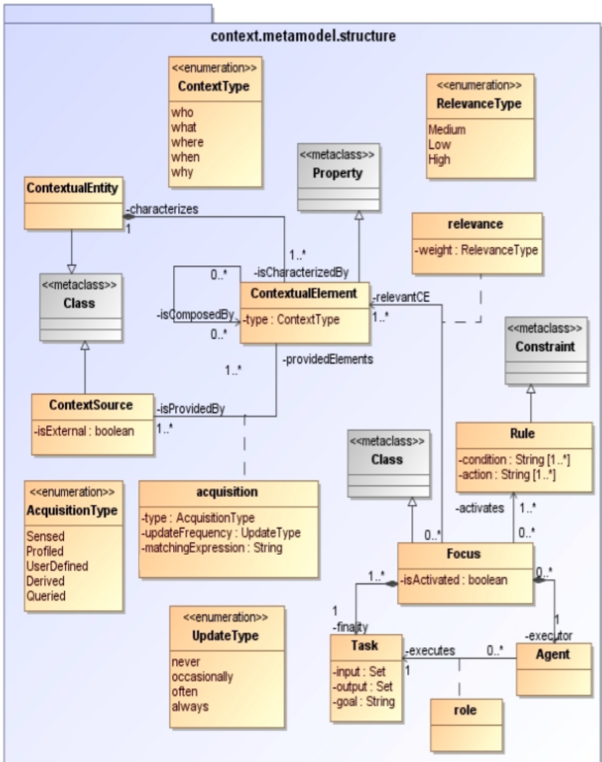
Figura 2.8 Metamodelo de contexto (Vieira, 2008)
