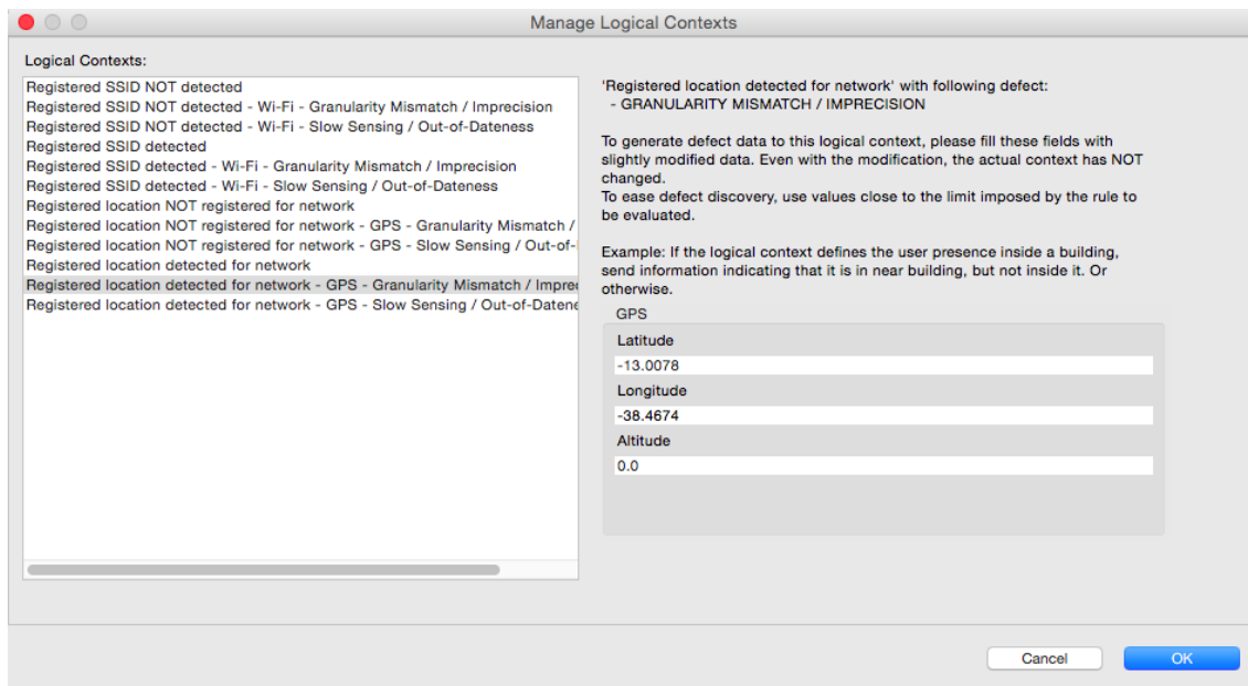
Figura 3.29 Execução da tarefa Identificar Contextos Lógicos na aplicação PersonalUpload-Manager . Destaque para a definição do contexto de localização registrada na aplicação com o padrão de defeito Granularidade Incompatível/Imprecisão no sensor de GPS.
