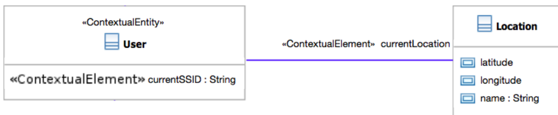
Figura 2.14 Diagrama com entidade contextual e elementos contextuais da aplicação PersonalUploadManager
