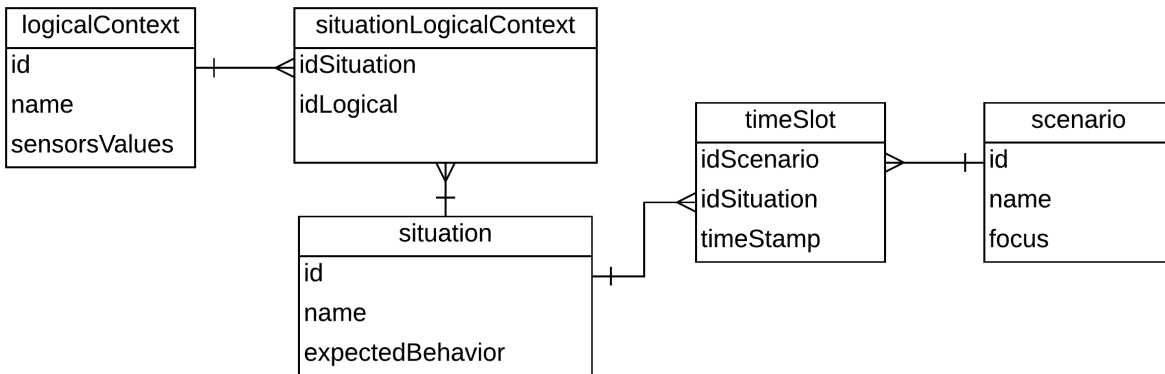
Figura 3.5 Diagrama de Entidade e Relacionamento da Base de Conhecimento de Contexto para Testes.
