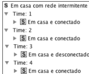
Figura 3.6 Cenário elaborado pelo testador. O cenário estrutura uma sequência de situações que indicam que o usuário está localizado em casa mas sua conectividade está intermitente. Este cenário é armazenado na CKTB e fica disponível para execução em diversos testes da aplicação.
