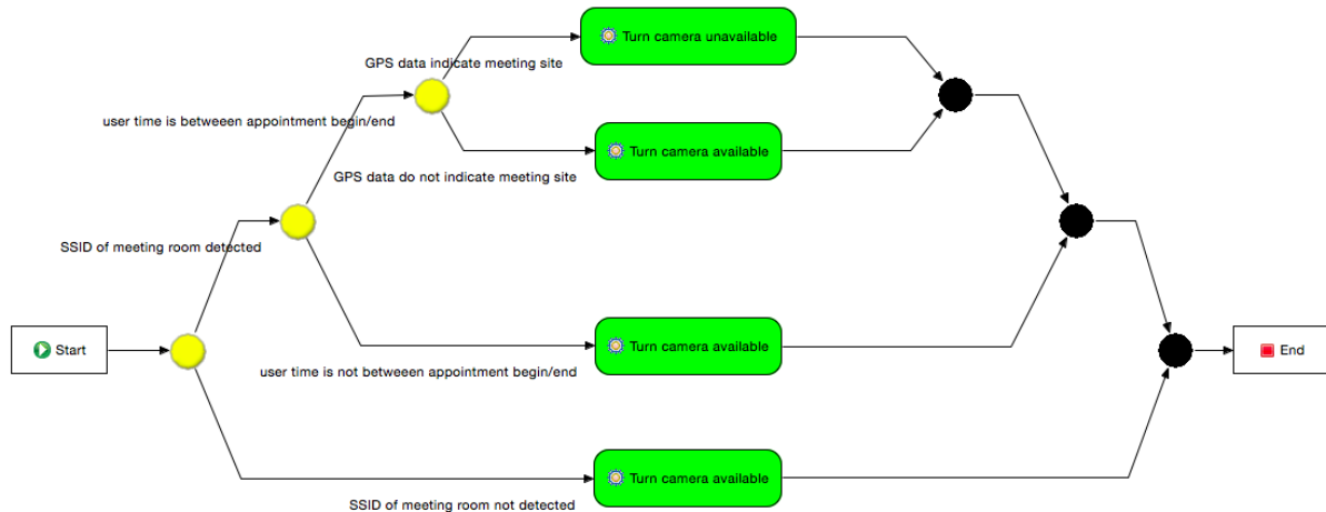
Figura 2.9 Grafo contextual de uma aplicação que gerencia a disponibilidade de uma câmera de acordo com o contexto do usuário.
