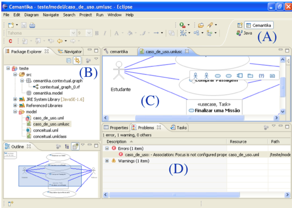
Figura 2.10 Modelagem de contexto com uso do metamodelo definido no framework CEManTIKA na ferramenta CEManTIKA Modeling (Patricio, 2010).
