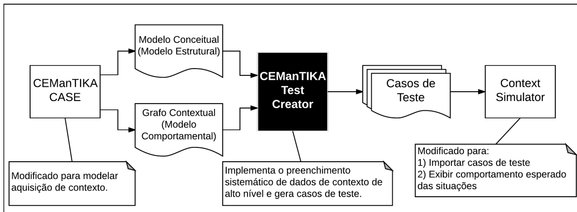
Figura 3.11 Visão geral da implementação do protótipo. Exibimos os ajustes feitos no CEManTIKA CASE, os modelos que são gerados e aproveitados como entrada para o CEManTIKA Test Creator, e os casos de teste que são gerados pelo CTC, os quais são executados por uma versão adaptada do Context Simulator.
