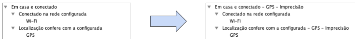
Figura 3.23 Exemplo de transformação de uma situação com o padrão de defeito Granularidade Incompatível/Imprecisão.
