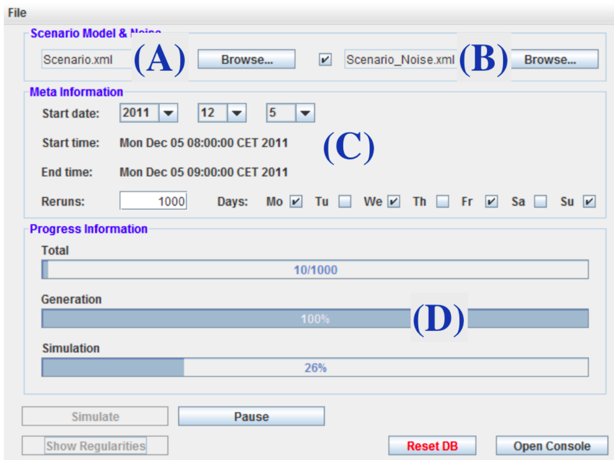
Figura 2.22 Protótipo do gerador de eventos de contexto que utiliza o formalismo DEVS. O protótipo implementado contempla também um simulador de contexto (Garzon e Hritsevskyy, 2012).
