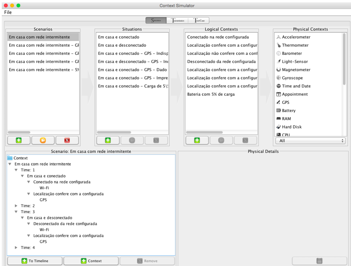
Figura 2.19 Exemplo de modelagem de um cenário. No cenário em destaque (Em casa com rede intermitente), cada intervalo de tempo (4 no total) contém uma situação, que pode ser “Em casa conectado” ou “Em casa e desconectado”. Cada situação pode ter contextos lógicos, e estes últimos são agregados com contextos físicos (sensores de GPS e Wi-fi).
