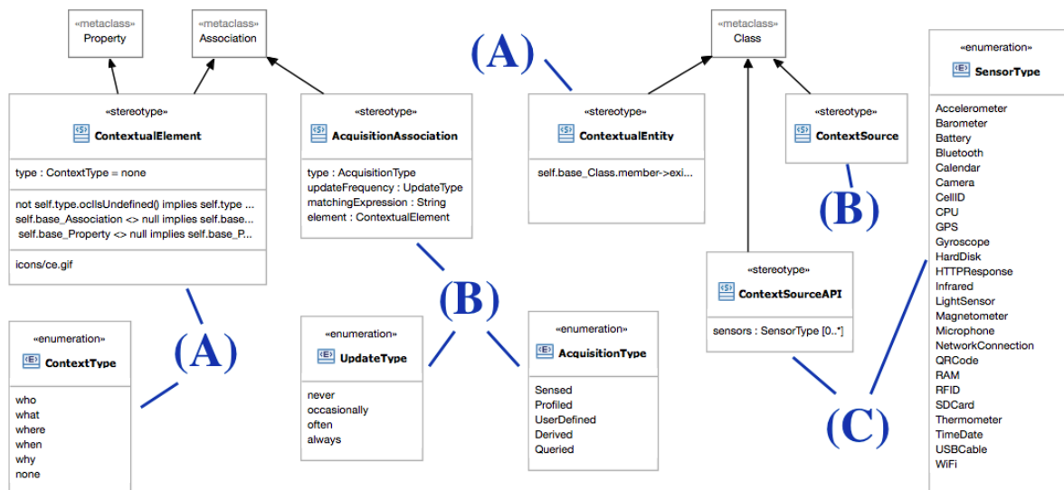
Figura 3.13 Metamodelo de contexto do CEManTIKA CASE. Os estereótipos associados a (A) são os originais da ferramenta CEManTIKA CASE, os que estão em (B) e (C) são frutos de ajustes na ferramenta. Os que estão associados a (B) já estavam previstos no framework CEManTIKA mas não estavam implementados na ferramenta, enquanto que os que se relacionam com (C) foram concebidos nesta dissertação.
