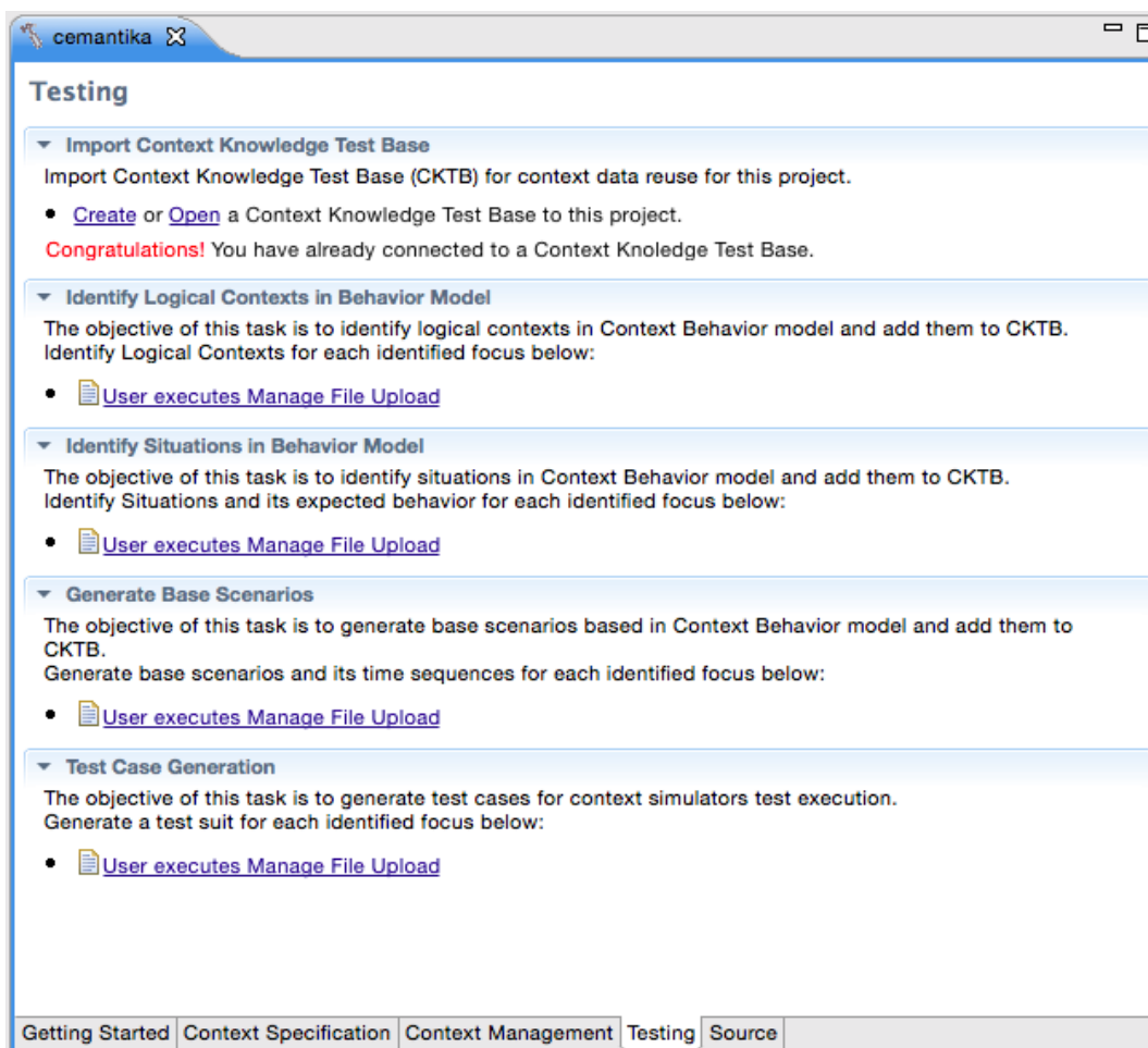
Figura 3.17 Implementação na ferramenta CEManTIKA CASE das tarefas de geração de casos de teste definidas no método CTC.
