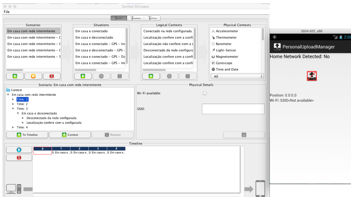
Figura 2.20 Execução de um cenário na aplicação exemplo. À esquerda temos o Context Simulator, e à direita temos a aplicação PersonalUploadManager sob teste. Os dados de contexto que estão destacados na linha do tempo são os enviados para o simulador de contexto no momento.
