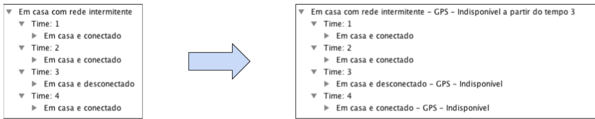
Figura 3.20 Exemplo de transformação do cenário da aplicação exemplo pelo padrão de defeito Incompleto/Indisponível, a partir do tempo 3.
