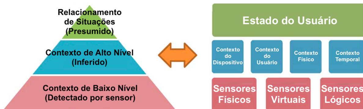
Figura 2.4 Pirâmide representando níveis de abstração de contexto segundo (Yürür et al., 2016)
