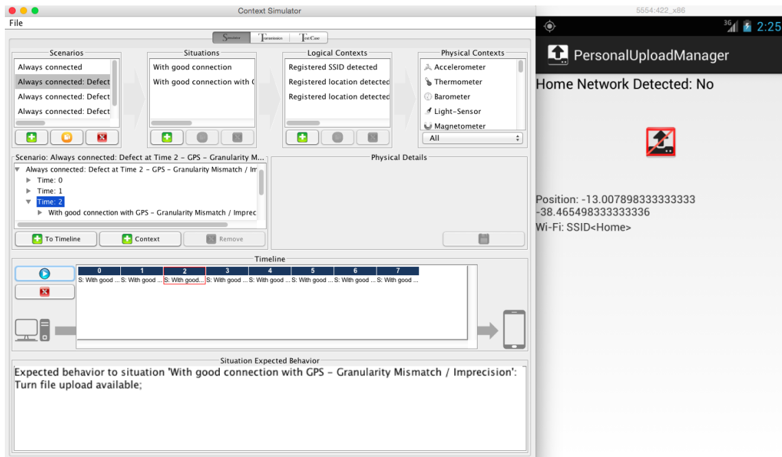
Figura 3.34 Aplicação sob teste com defeito descoberto após leitura de coordenada de GPS imprecisa presente no caso de teste executado.
