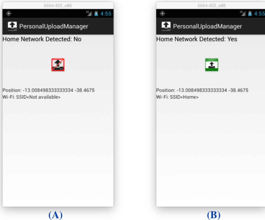
Figura 3.1 Aplicação PersonalUploadManager gerenciando o envio de dados do dispositivo. Na captura de tela à esquerda (A), a aplicação não reconhece o contexto de uma conexão configurada pelo usuário e bloqueia o envio de dados. Na tela à direita (B), o aplicativo reconhece o contexto de uma conexão de dados configurada pelo usuário e libera o envio de dados pelo dispositivo.
