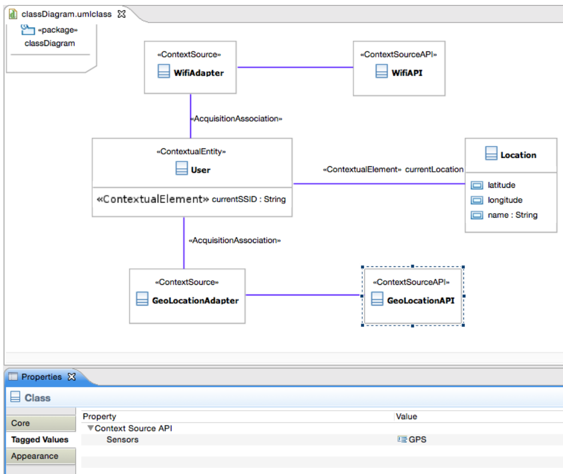
Figura 3.14 Diagrama com especificação de aquisição de contexto e das API's de fontes de contexto da aplicação PersonalUploadManager . Destaque para a especificação do sensor de GPS para a API de fonte de contexto GeoLocationAPI , a qual fornece dados de contexto para o elemento contextual de localização do usuário.
