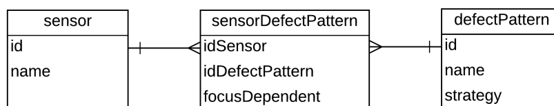
Figura 3.7 Diagrama de Entidade e Relacionamento do Repositório de Padrões de Defeitos de Contexto.
