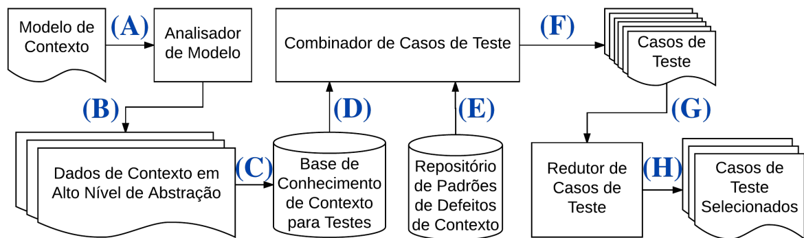
Figura 3.2 Componentes da arquitetura proposta
