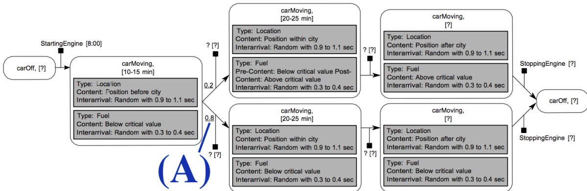
Figura 2.21 Cenário de uso típico de uma aplicação cujo foco é a emissão de alertas para motoristas em um percurso (Garzon e Hritsevskyy, 2012)
