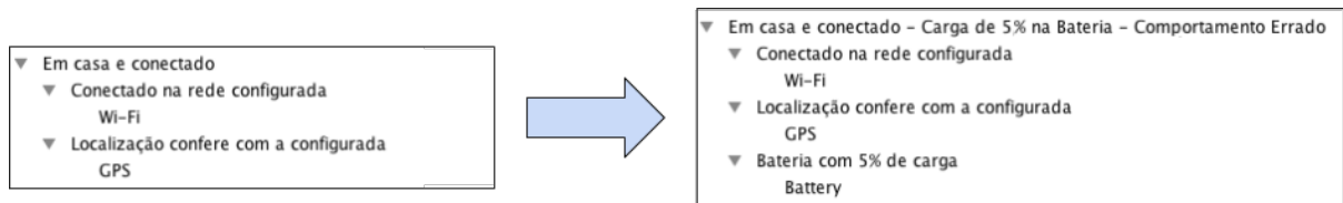
Figura 3.25 Exemplo de transformação de uma situação com o padrão de defeito Regra Lógica Problemática/Comportamento Errado Causado por Interrupções.
