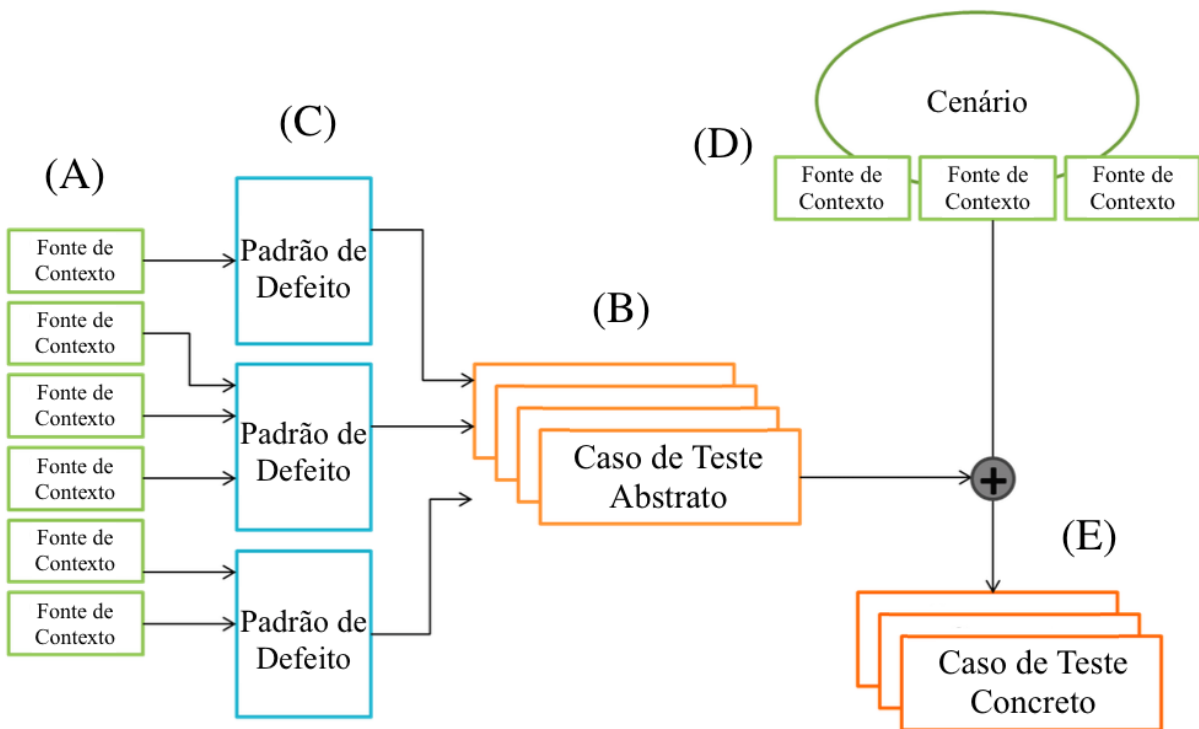
Figura 2.7 Relação entre os padrões de defeitos em fontes de contexto e os artefatos de teste, como casos de teste abstratos e concretos (Hassel, 2014)
