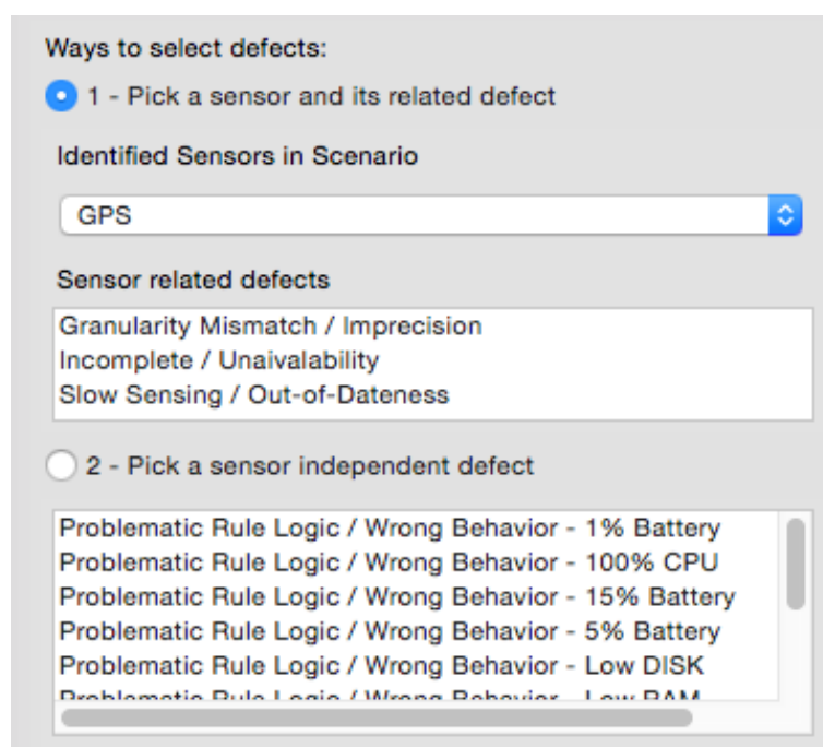
Figura 3.27 Escolhendo padrões de defeitos para gerar os casos de teste na ferramenta CEManTIKA CASE.
