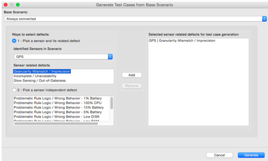
Figura 3.32 Execução da tarefa Combinar Cenários Base com Padrões de Defeitos na aplicação PersonalUploadManager . O testador combina o cenário em que o usuário está com o contexto que libera a funcionalidade de enviar dados com o padrão de defeito Granularidade Incompatível/Imprecisão no sensor de GPS.
