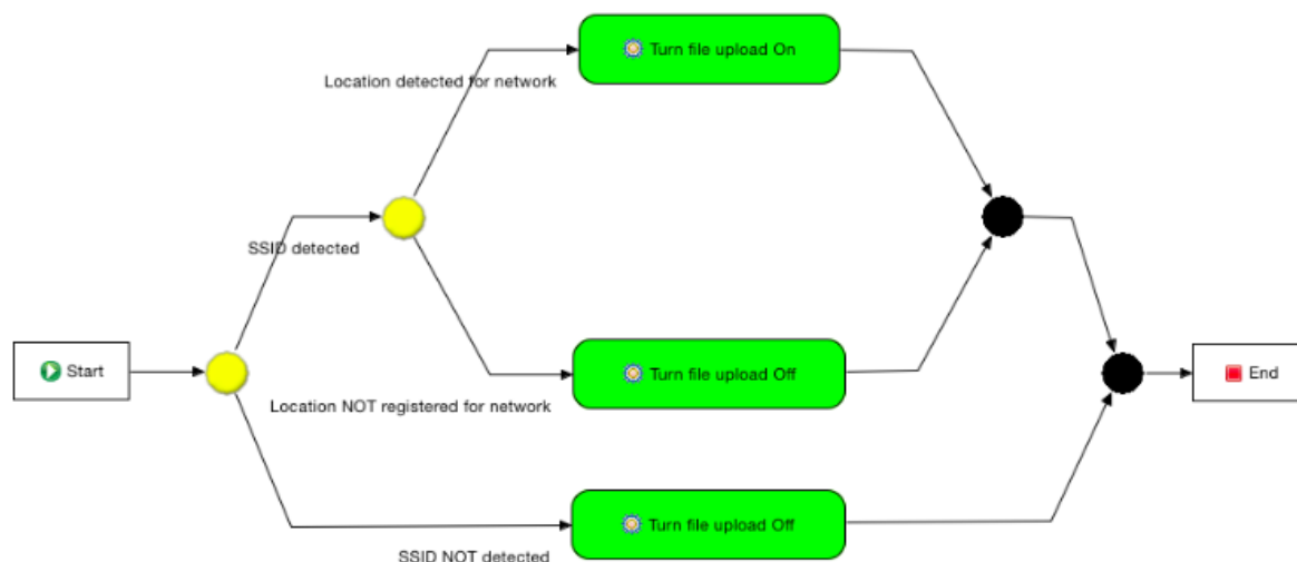
Figura 3.18 Modelo comportamental de contexto da aplicação PersonalUploadManager seguindo grafo contextual do metamodelo CEManTIKA.
