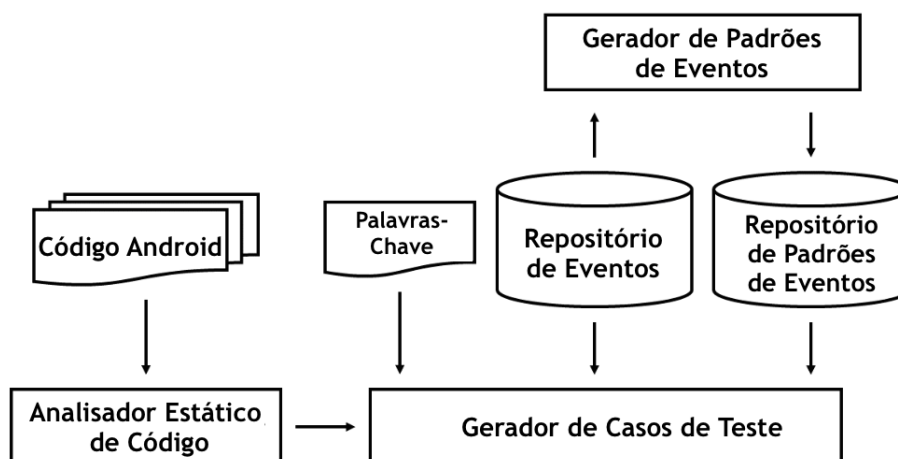
Figura 2.23 Arquitetura de uma solução que gera casos de teste a partir de código-fonte de aplicações Android, com uso de padrões de eventos de contexto (Yu e Takada, 2015)
