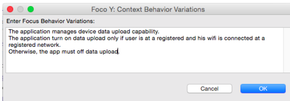
Figura 2.13 Tela do CEManTIKA CASE onde o projetista identifica as variações de comportamento de um foco.
