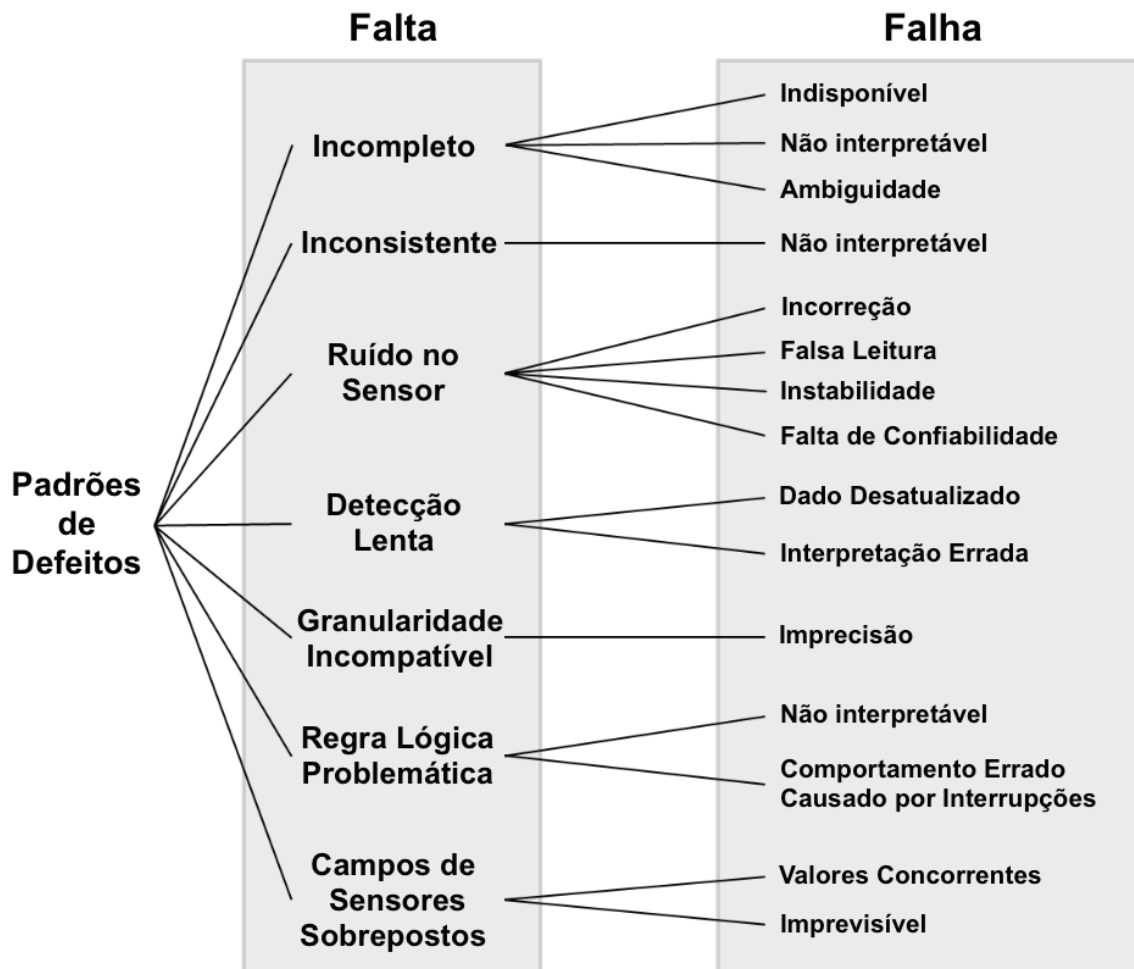
Figura 2.6 Padrões de defeitos que podem afetar sensores físicos em um aplicativo móvel (Hassel, 2014), adaptado de (Sama et al., 2008).
