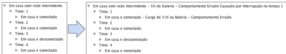
Figura 3.26 À esquerda, o cenário escolhido. À direita, o cenário derivado após aplicação do Padrão de defeito Regra Lógica Problemática/Comportamento Errado Causado por Interrupções para indicar que a bateria atingiu 5% de carga no tempo 1.
